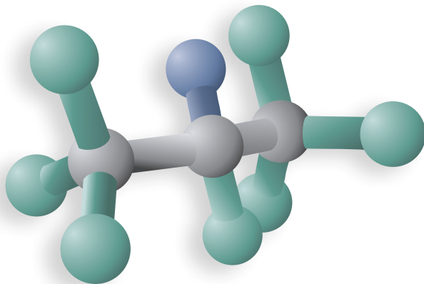
HFC-227ea Molekül
